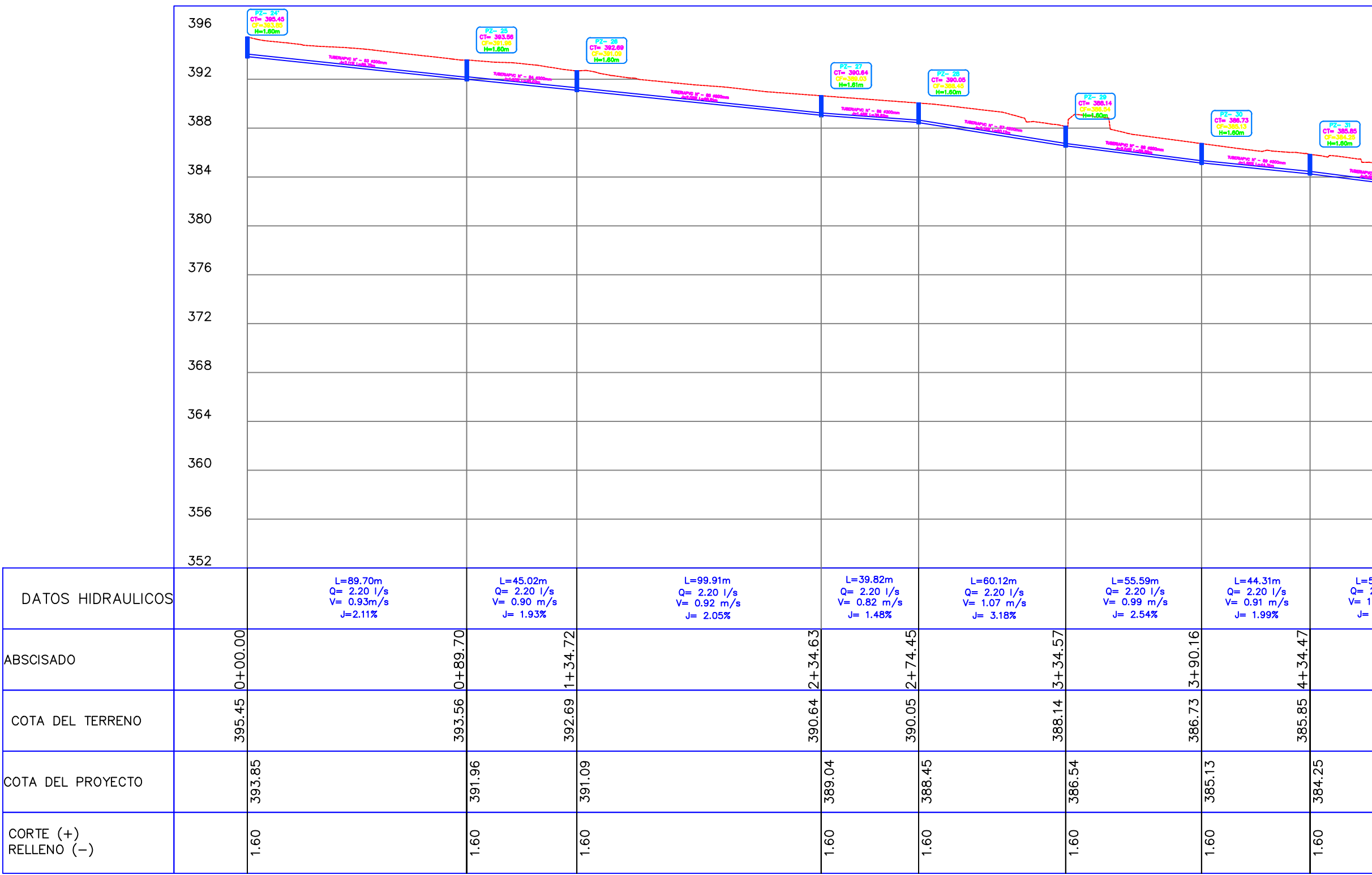
PERFIL LONGITUDINAL CALLE 3 H: 1/1000 V: 1/200
